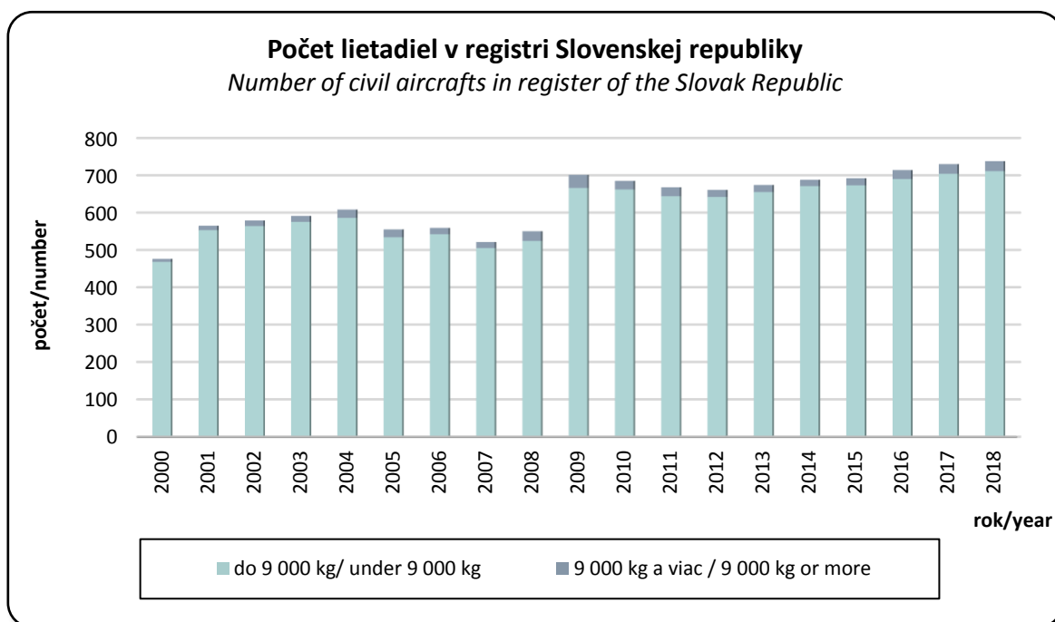
GRAF 9 POČET LIETADIEL V REGISTRI SLOVENSKEJ REPUBLIKY GRAPH 9 NUMBER OF CIVIL AIRCRAFTS IN REGISTER OF THE SLOVAK REPUBLIC (GRAFICKÉ ZNÁZORNENIE TABUĽKY 4.4) (GRAPHIC REPRESENTATION OF TABLE 4.4)
